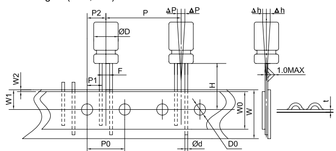
Drawing IV (Ø16,Ø18)
